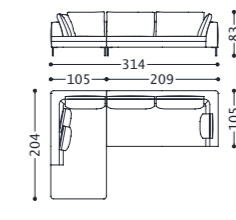
01CL2C4 (1CL2CHLSX - 1CL2D2MDX) 02CL2C4 (2CL2CHLSX - 2CL2D2MDX)
